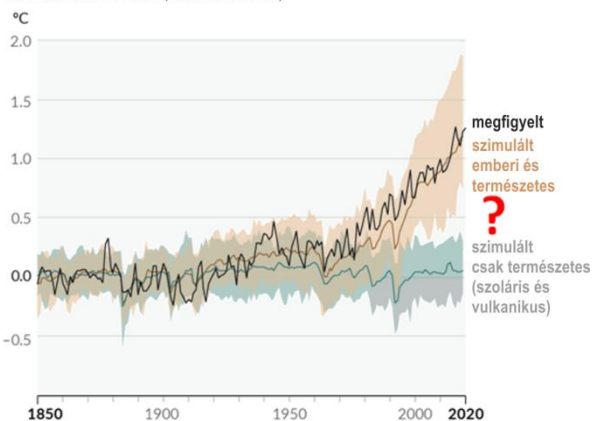
4. ábra. Az IPCC AR5 WG1 SPM.1 ábra: (a) a globális átlagos felszínhőmérséklet-anomália időbeli változása rekonstrukció alapján (1-től 2000-ig) és mérések alapján (1850-től 2020-ig); (b) a globális átlagos felszínhőmérséklet-anomália alakulása mérés és modellezés alapján (1850-től 2020-ig). A kék szín az IPCC által kizárólag a természetnek tulajdonított változást mutatja, míg a barna szín a természeti és az emberi hatásokat együttesen [23]
