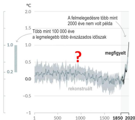
4. ábra. Az IPCC AR5 WG1 SPM.1 ábra: (a) a globális átlagos felszínhőmérséklet-anomália időbeli változása rekonstrukció alapján (1-től 2000-ig) és mérések alapján (1850-től 2020-ig); (b) a globális átlagos felszínhőmérséklet-anomália alakulása mérés és modellezés alapján (1850-től 2020-ig). A kék szín az IPCC által kizárólag a természetnek tulajdonított változást mutatja, míg a barna szín a természeti és az emberi hatásokat együttesen [23]
